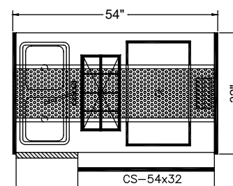
CS-54x32-CCW (plan view)
