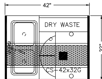
CS-42x32G-CW (plan view)
