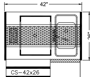
CS-42x26-CW (plan view)
