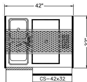
CS-42x32-CCW (plan view)
