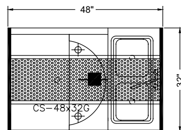
CS-48x32G-CCW (plan view)
